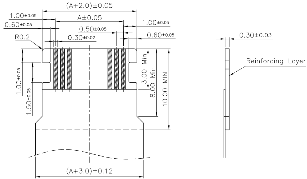
PCB LAYOUT(正脚)
