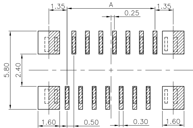
PCB LAYOUT(正脚)
